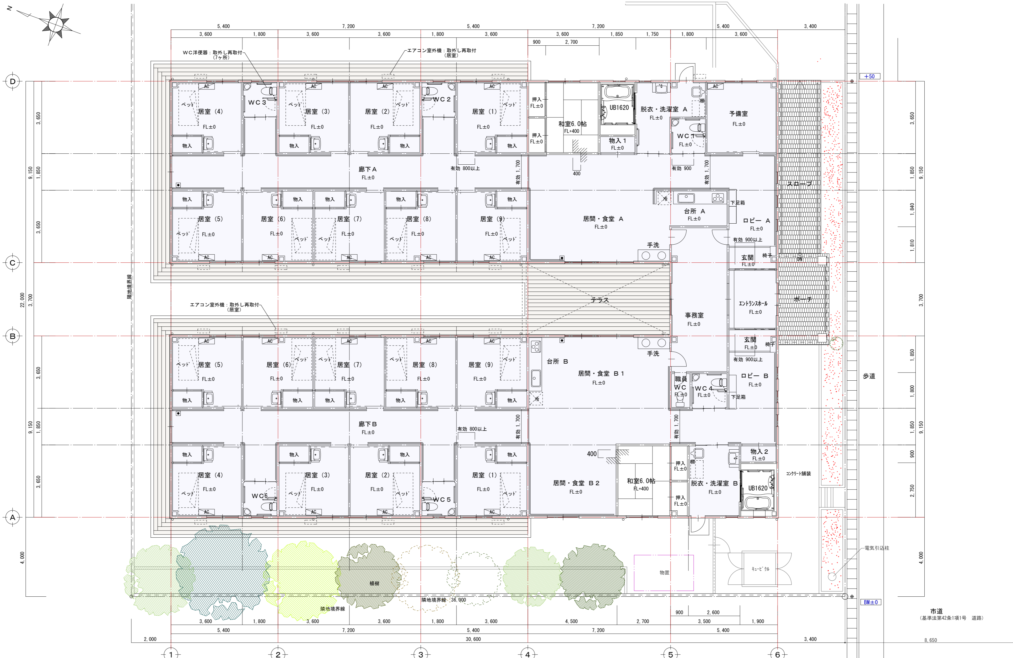
1階平面図 S=1/100
